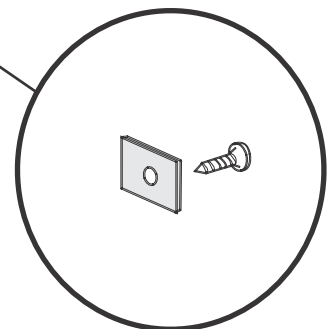
Distantier plastic folosit in cazul tamplariilor cu inclinatie mai mare de 5 grade.
