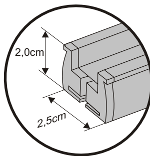
Profil superior si inferior din aluminiu Culori: ALB
