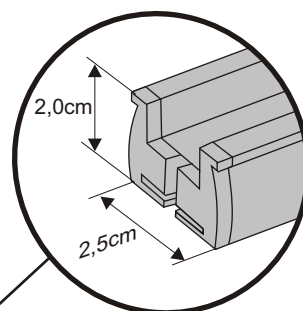
Profil superior si inferior din aluminiu Culori: ALB si NEGRU
