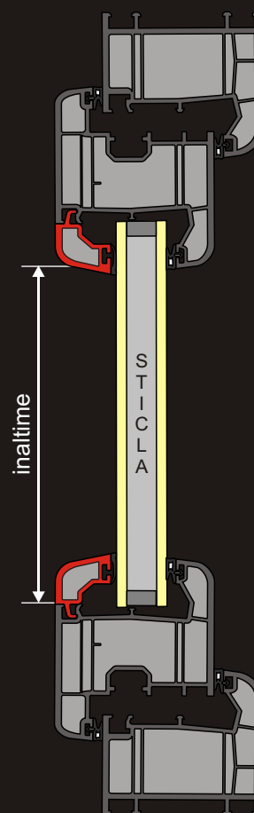
Detaliu preluare cota pentru inaltime
