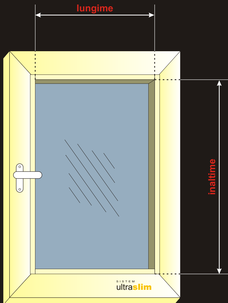
Detaliu preluare cota pentru lungime tamplarie cu bagheta rotunjită
