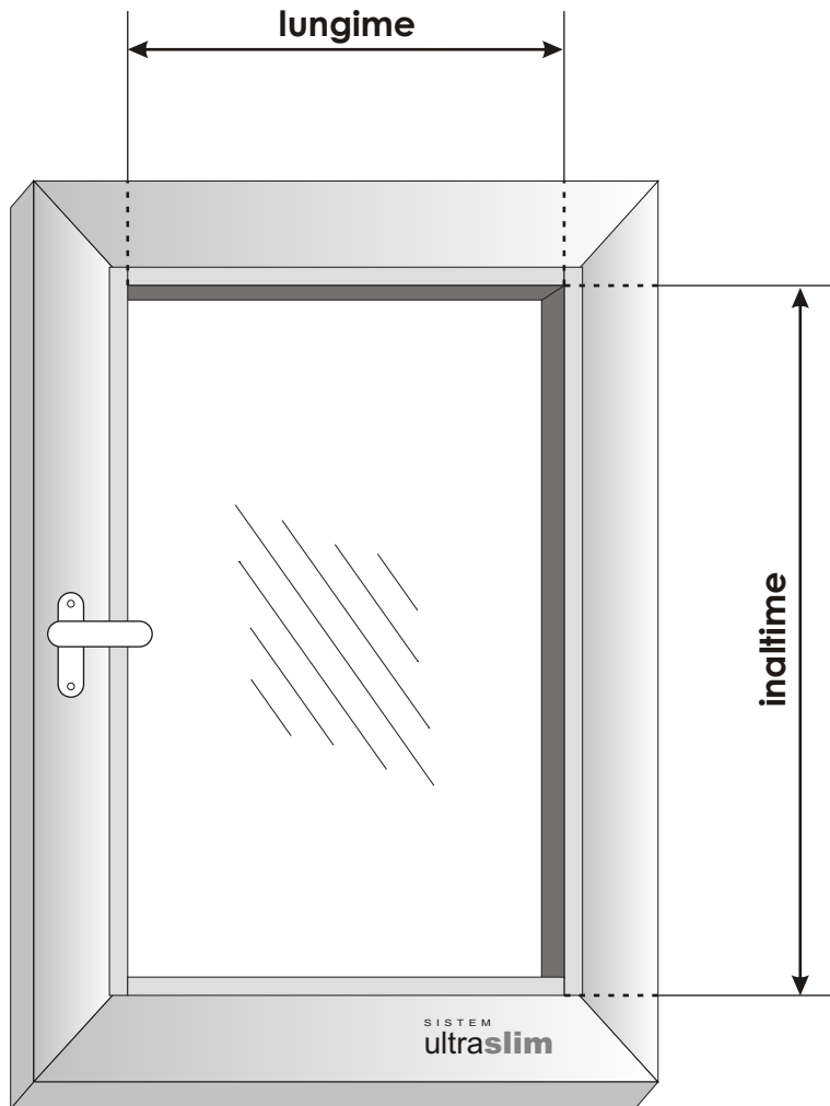
Detaliu preluare cota pentru lungime tamplarie cu bagheta rotunjita
