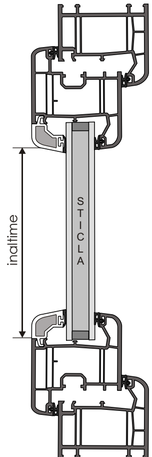
Detaliu preluare cota pentru inaltime
